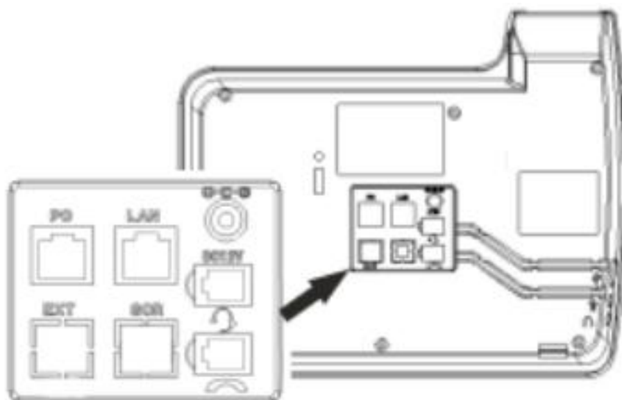
图 2.1 ES330-PES 话机背部连接接口
